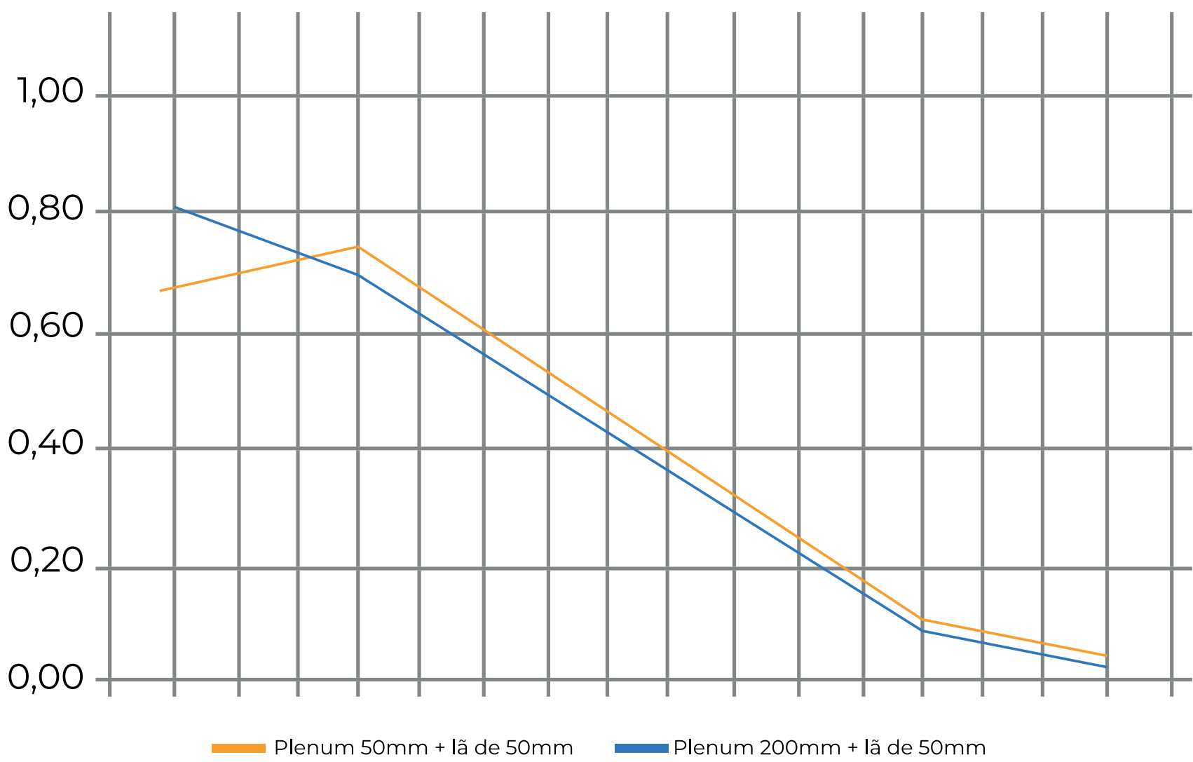
Gráfico - Curva Coeficiente de Absorção Sonora
